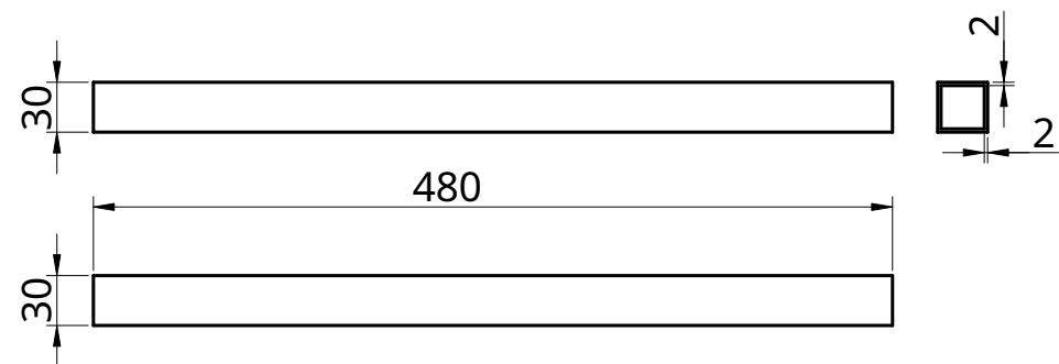
TRAVERSE INFERIEURE 1:5
