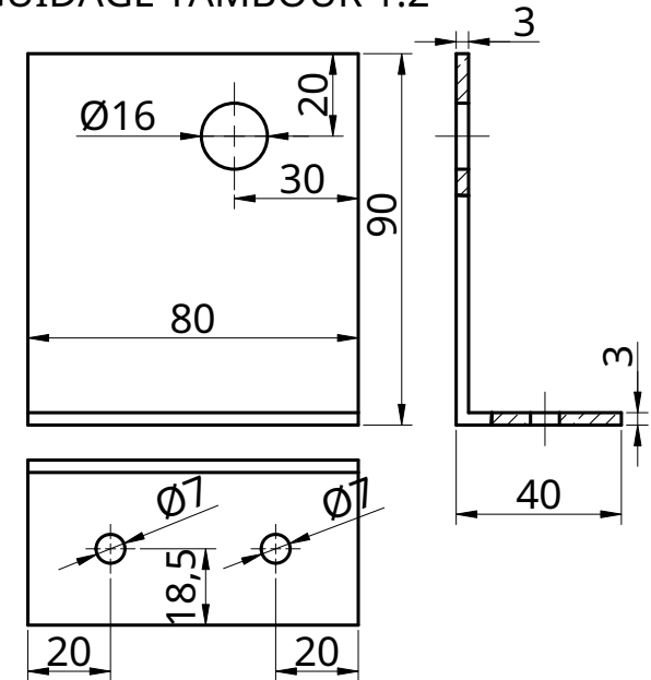
GUIDAGE TAMBOUR 1:2
