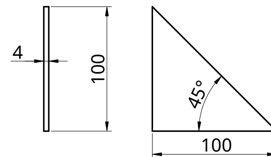
EQUERRE 1:3
