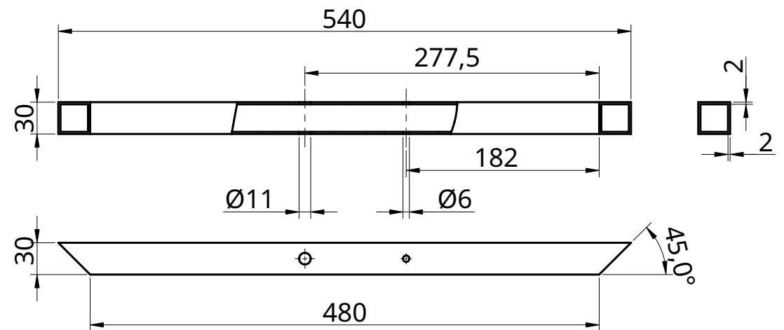
TRAVERSE SUPERIEURE 1:5
