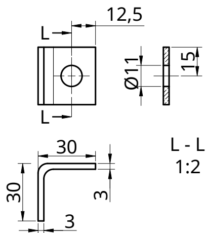
SUPPORT ROULEMENT 1:2
