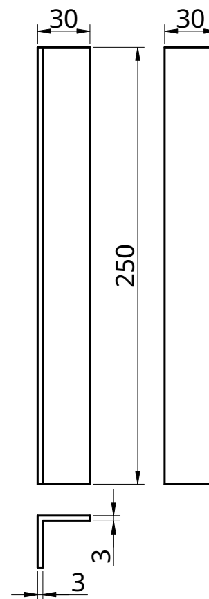
RENFORT VERTICAL 1:3
