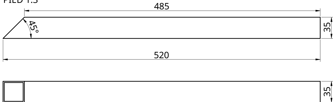
PIED 1:3
