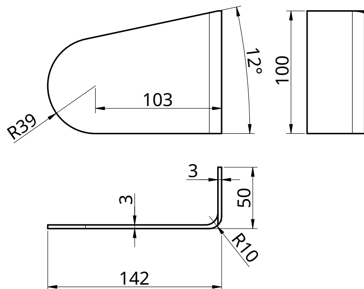
SUPPORT DE ROUE 1:3
