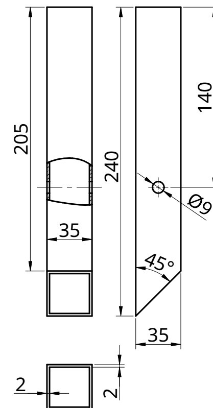
MANCHON 1:3
