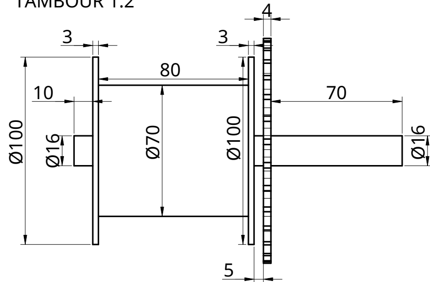
TAMBOUR 1:2
