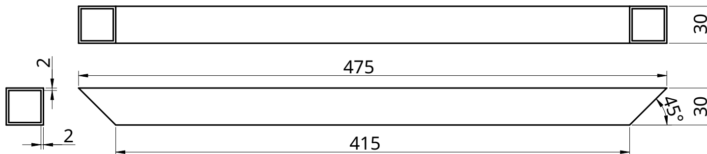
BARRE HORIZONTALE 1:3
