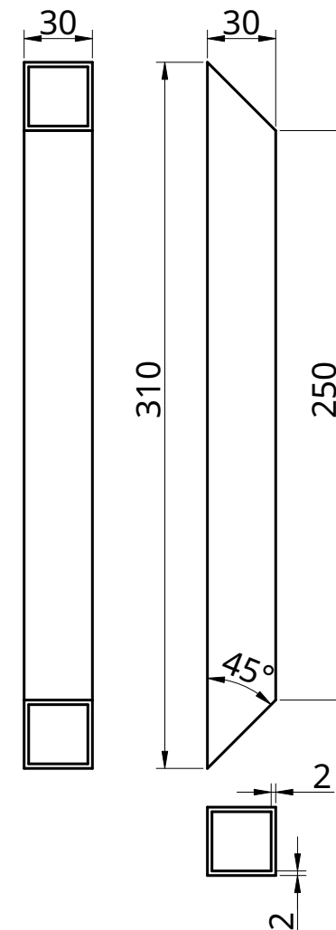
BARRE VERTICALE 1:3
