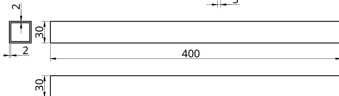
FOURCHE 1:3
