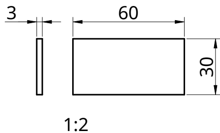
BUTEE 1:2
